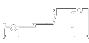
OP161 Sill
