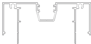
OP160 Jamb
