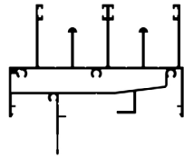
Sill / Transom
