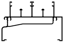
Sill / Transom
