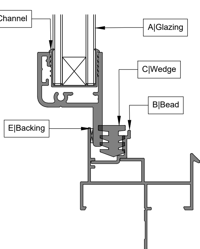
CSW3 Jamb CSW12 Bead
