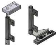
Std. R/H Pivot Set 93-103C
